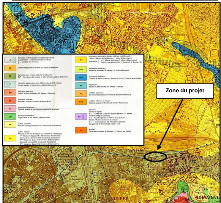
Extrait de la carte géologique de Paris au 1/25 000 ème
